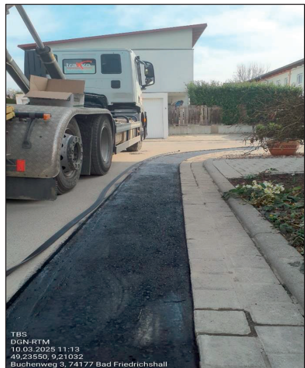
Asphalttragschicht eingebaut
