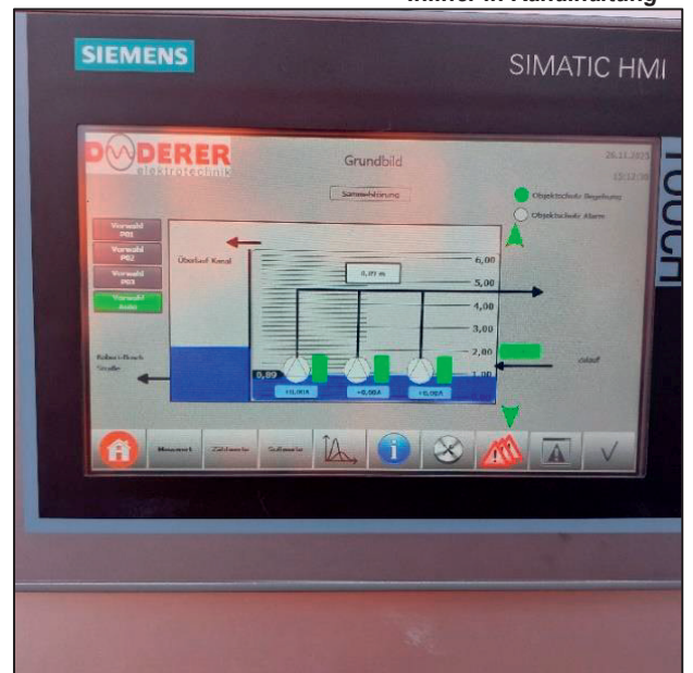
Fernwirktechnik Display vor Ort Damaschkestr.
