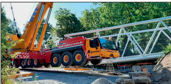
Einhub Brückenteil
