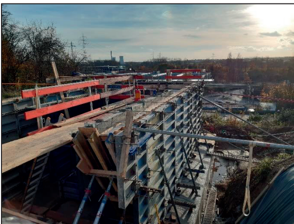
Widerlager am Radweg
