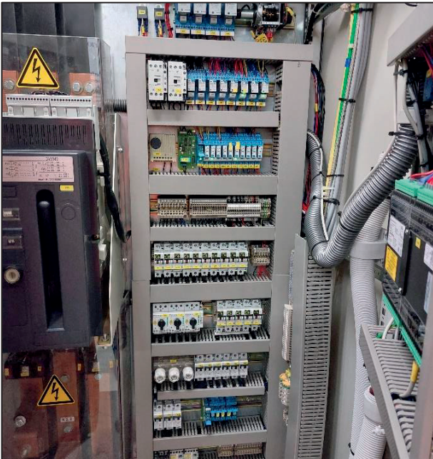
Schaltschrank Notstromaggregat neu
